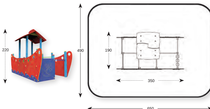
MÉRETEK + BIZTONSÁGI ZÓNA
