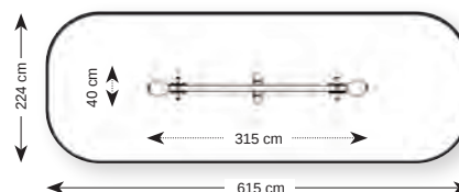
MÉRETEK + BIZTONSÁGI ZÓNA
