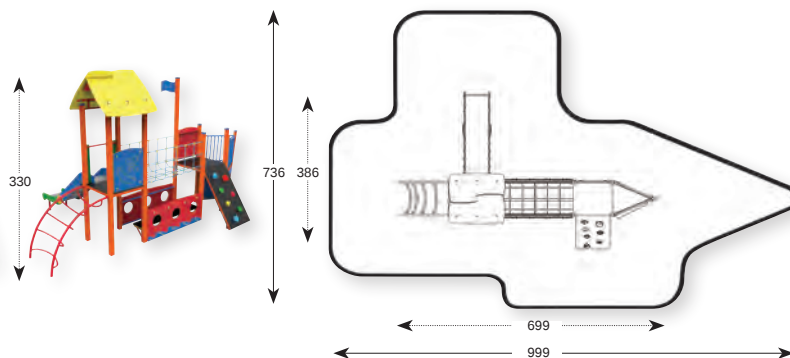
MÉRETEK + BIZTONSÁGI ZÓNA
